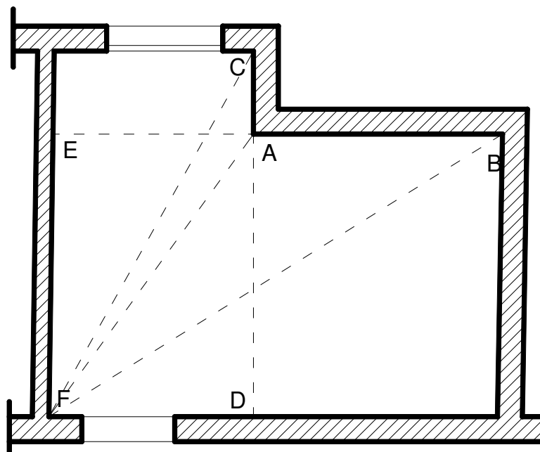
Figure 22: le relevé d'un décrochement
